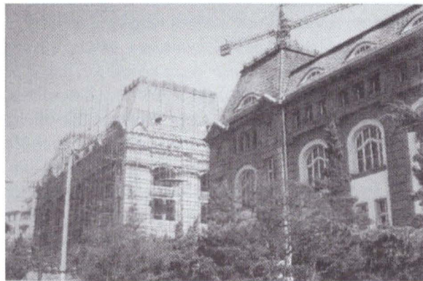
Der westliche Flügel des ehem. deutschen Gouvernment-Dienstgebäudes und sein „Spiegelbild“ im Bau, Qingdao März 1989
